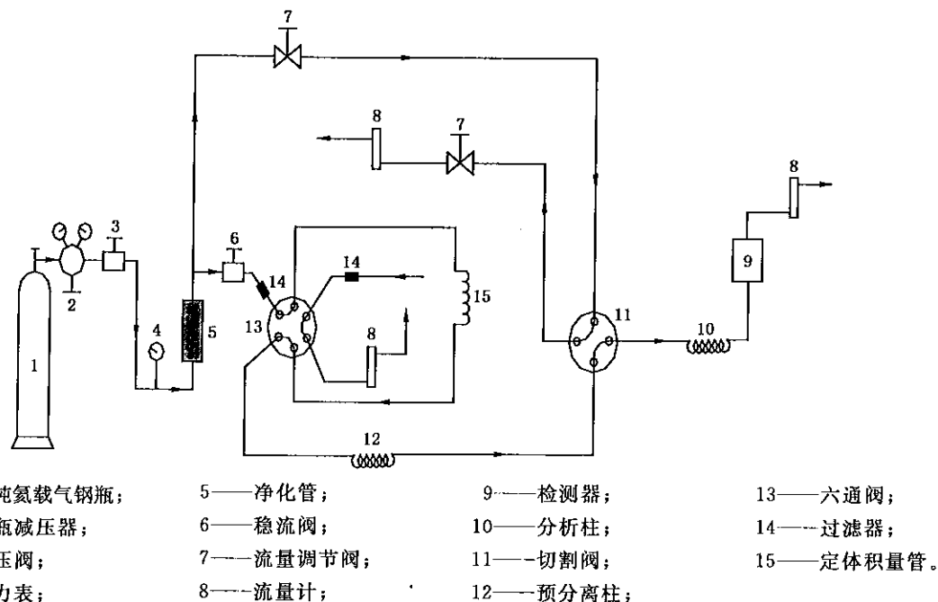
图 A.1 切割气路流程示意图
